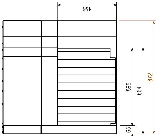
Front aanzicht
